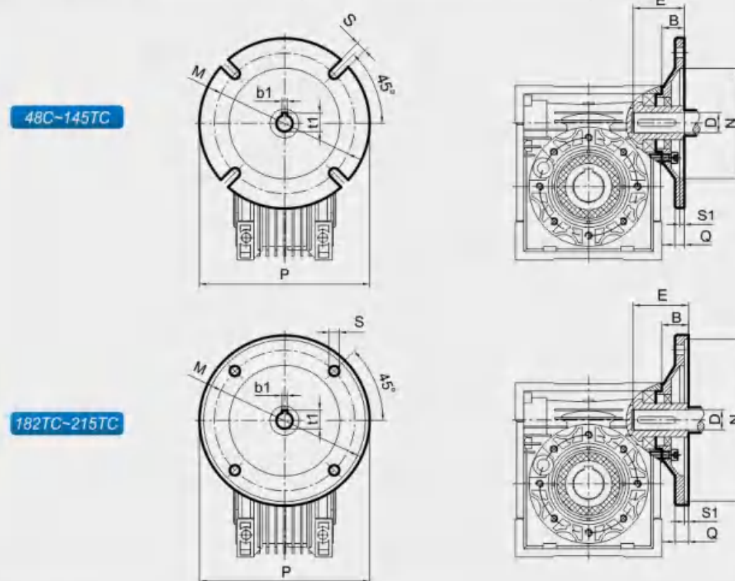
NMRV..NEMA输入法兰尺寸 / Input Flange Dimension
