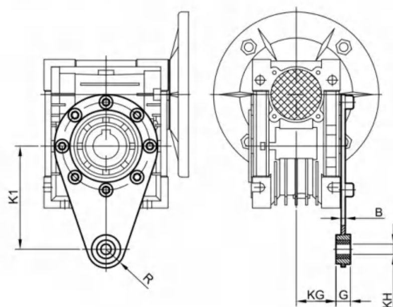
扭力臂 / Torque Arm
