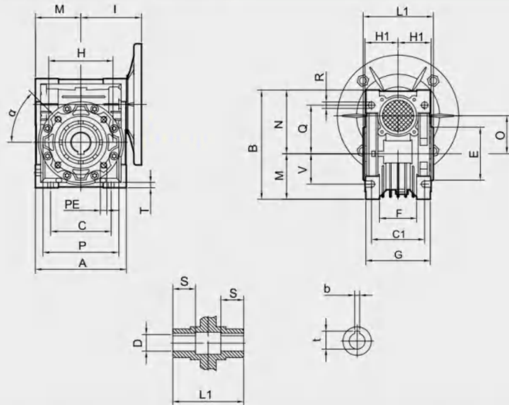
NMRV外形尺寸 / NMRV Outline Dimension
