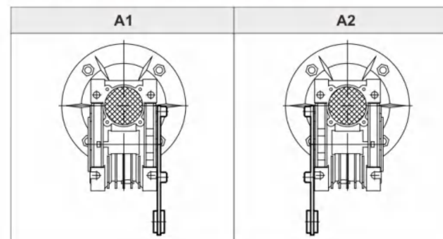
扭力臂 ( A ) 位置 / Torque arm (A) position
